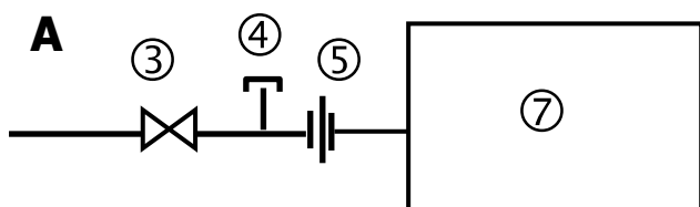
Chaudière sans vanne intégrée
